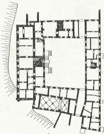
Zamek w Otmuchowie 1:1000
