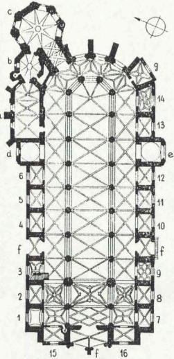
Kościół par. św. Jakuba w Nysie 1:75
