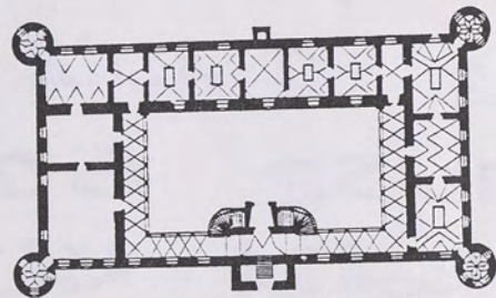
Rys. 66. Baranów. Zamek (1591—1606). Plan. 1 : 750
