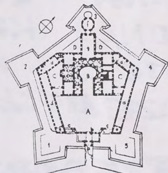
Zamek «Krzyżtopór» w Ujeździe 1:2000 (I. piętro)
