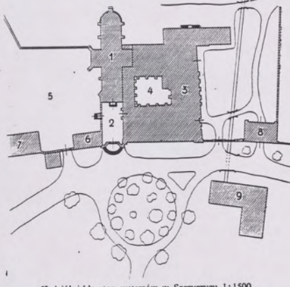
Kościół i klasztor cystersów w Szczyrzyku 1:1500
